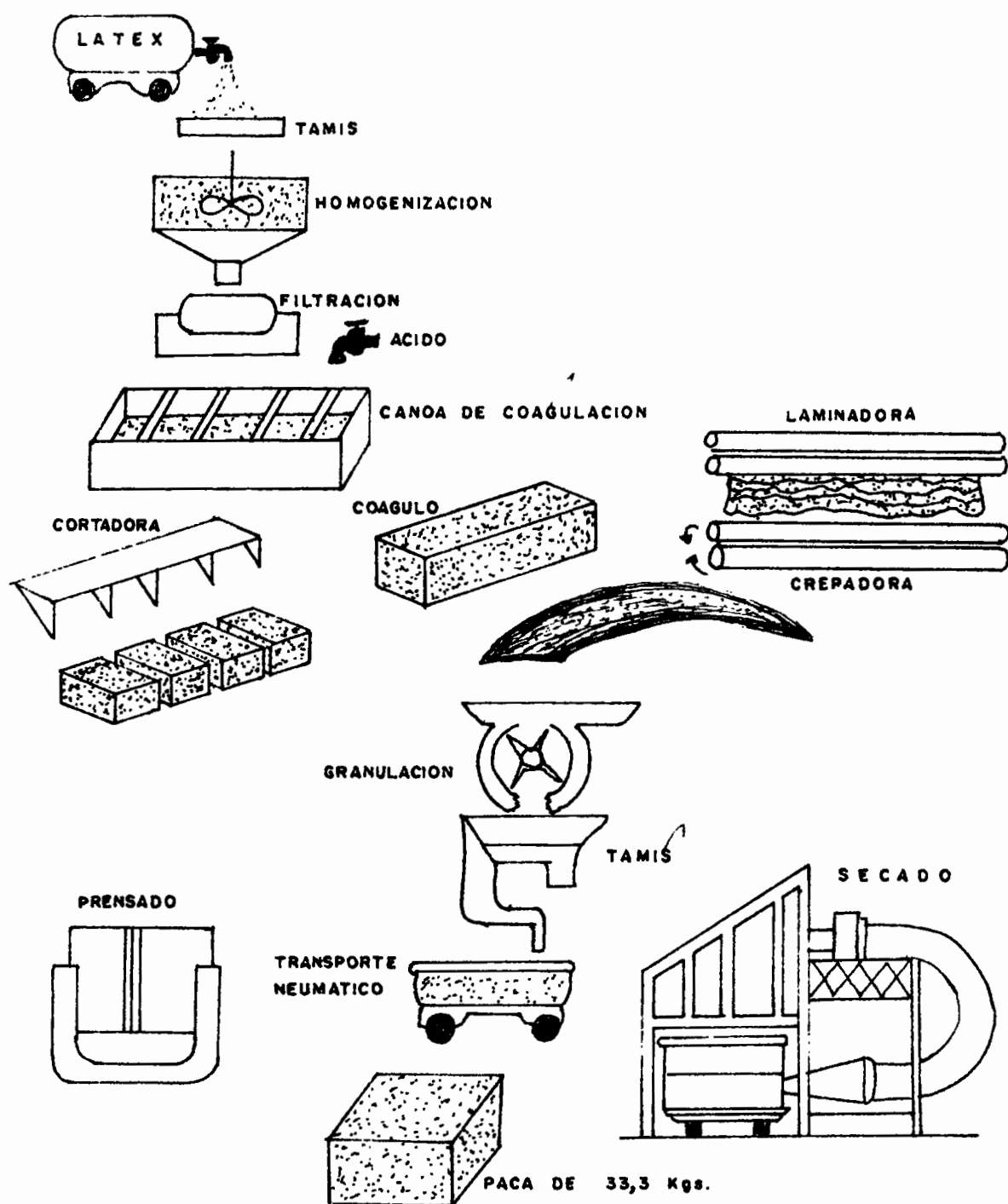
Fig. 11 ESQUEMA GENERAL DE LA PRODUCCION DE CAUCHO GRANULADO
